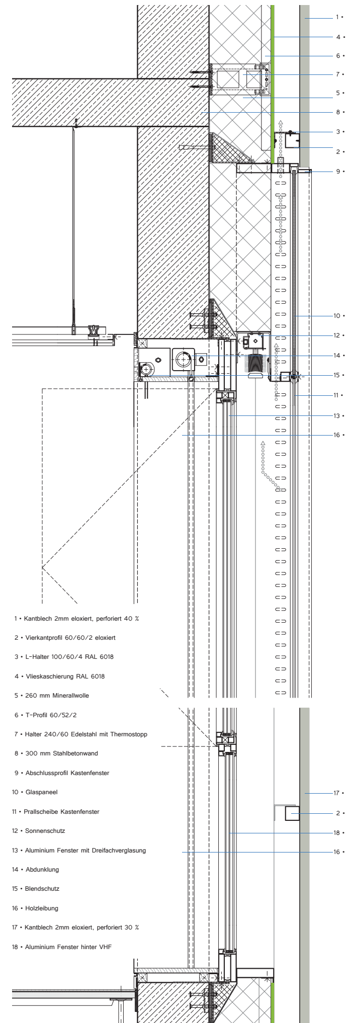
Fassadenschnitt
